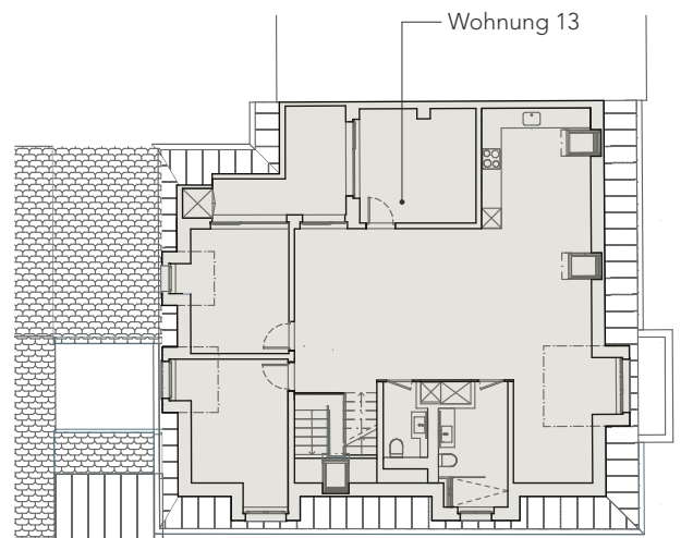
5. Obergeschoss
