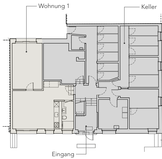
Erdgeschoss
